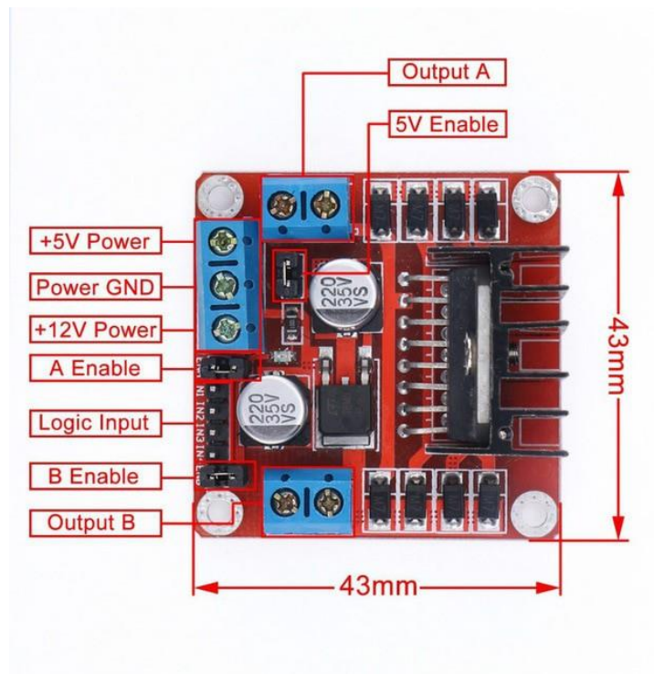
ภาพ 2.18 L298N Motor Drive
