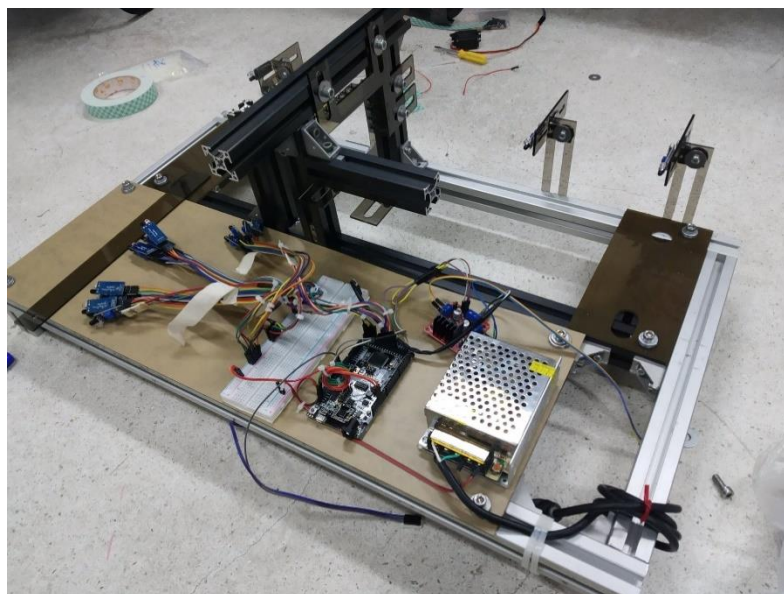
ภาพ 3.27 จัดระบบไฟฟ้าให้เป็นระเบียบเรียบร้อย
