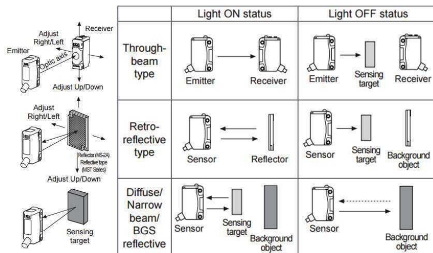
ภาพ 2.1 Photoelectric Sensor
