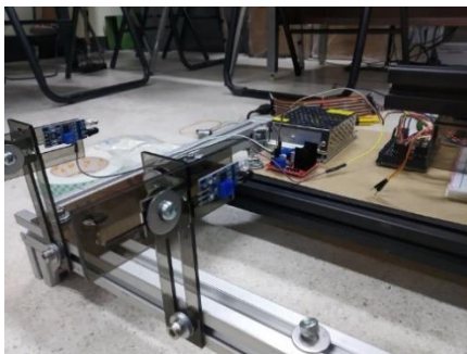
ภาพ 3.26 การต่อเซนเซอร์
