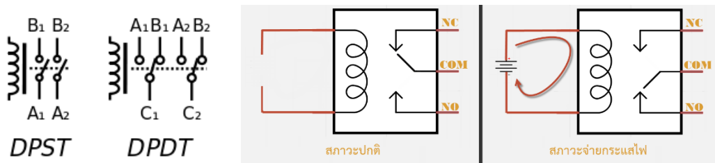
ภาพ 2.22 SPDT- Single Pole Double Throw
